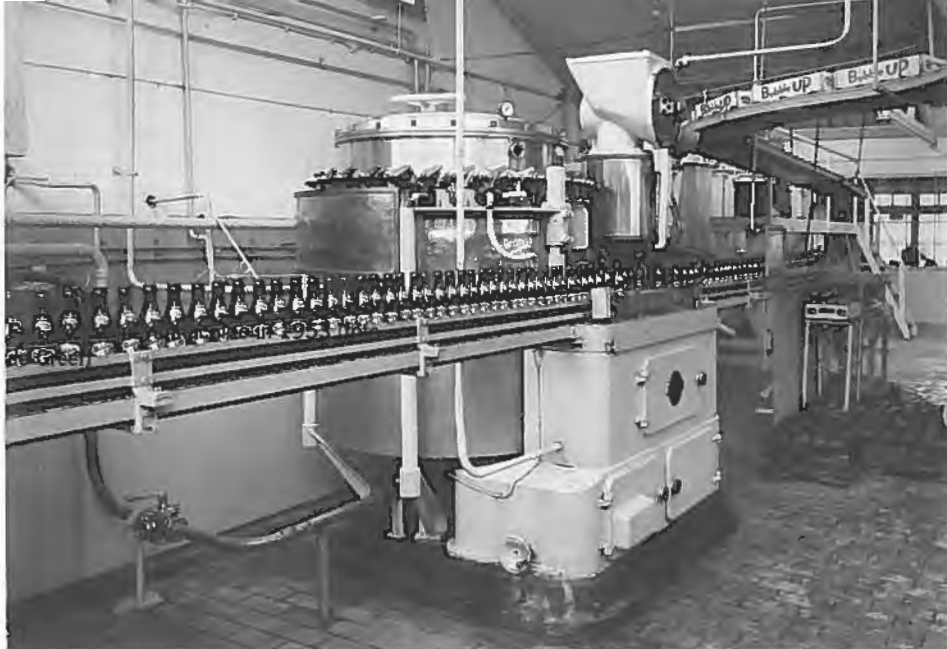
Een 30-kraansvulmachine in 1953 (foto de Greef)
