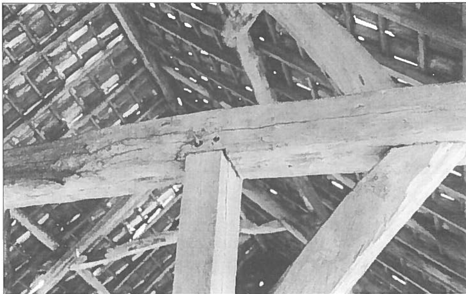
Afbeelding 5 Deel van de houtconstructie van de open loods.
