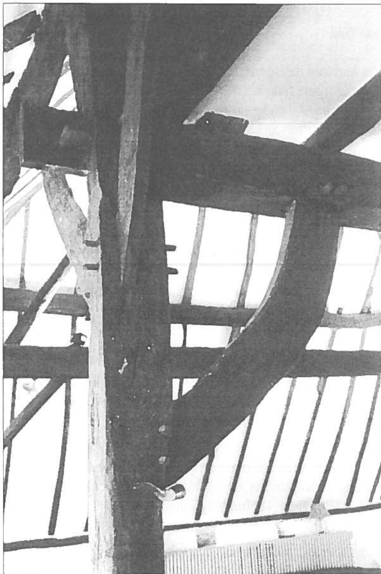
Deel van het gebint met stijl, ankerbalk en korbelen
