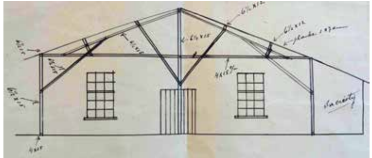
Bouwtekening van de voorgevel. BHIC Den Bosch, 156 nr. 90
