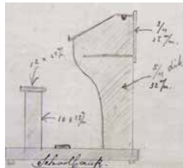
Schets van de schoolbanken volgens offerte van Louis Rombouts.
